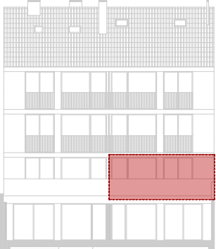
ALÇADO TARDOZ
