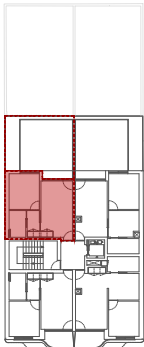
PLANTA GERAL
